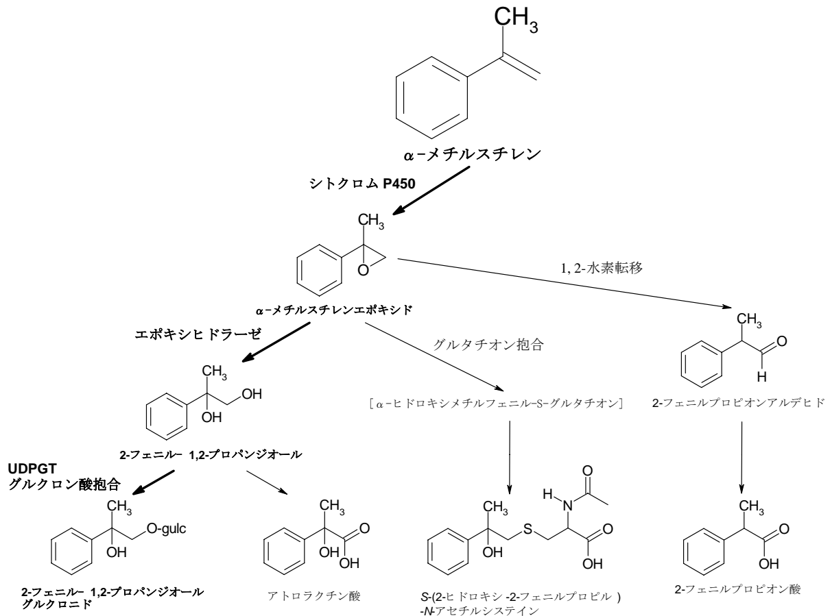
図 7-1 α-メチルスチレンの代謝経路図（出典：De Costa et al., 2001）
