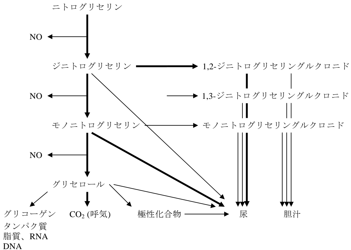
図 7-1 ニトログリセリンの代謝経路図
