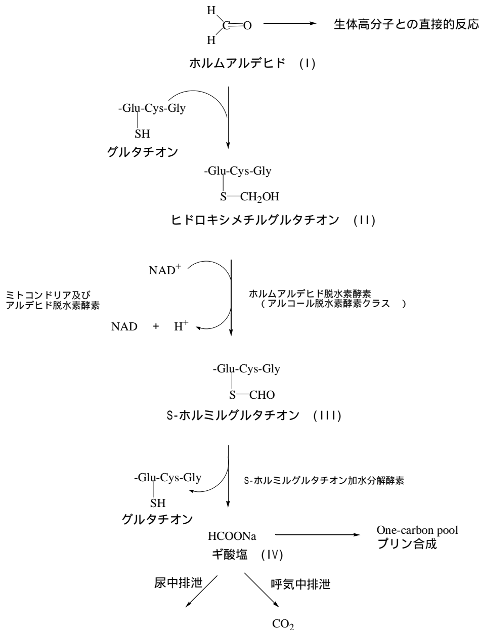
図 7-1 ホルムアルデヒドの代謝経路 (IPCS, 1989; IARC, 1995)
