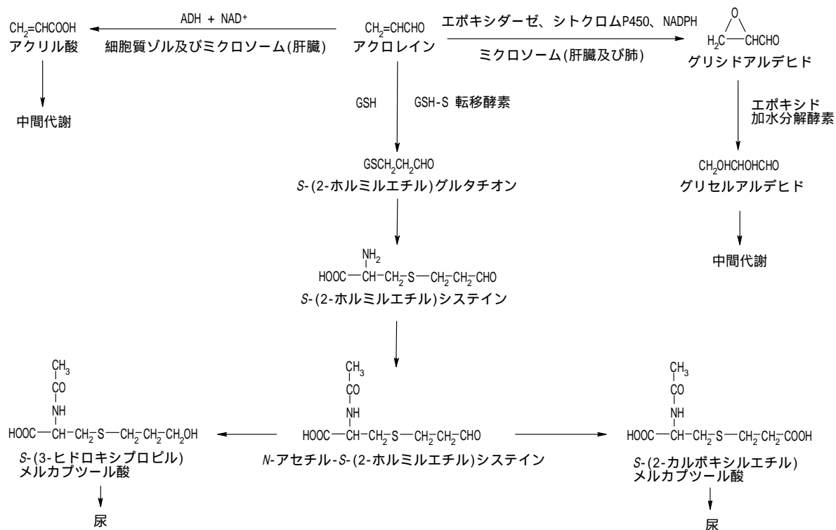
図 7-1 アクロレインの代謝経路図 (IPCS, 2002)
