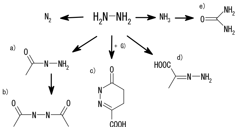
図 7-1 ヒドラジンの代謝経路 (Preece et al., 1991による)
