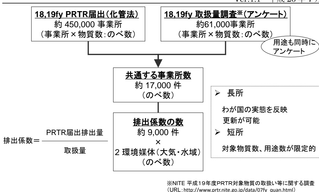
図表 IV-70 PRTR データ等からの排出係数の算出フロー
