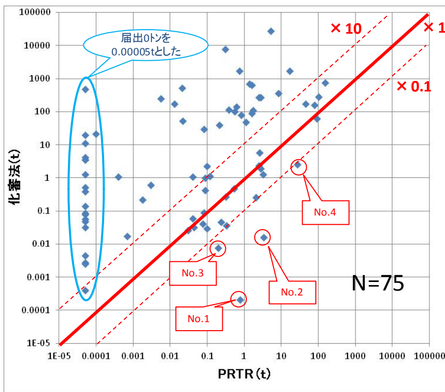
図表 IV-129 化審法推計排出量と PRTR 届出排出量最大排出源の比較検証—水域
