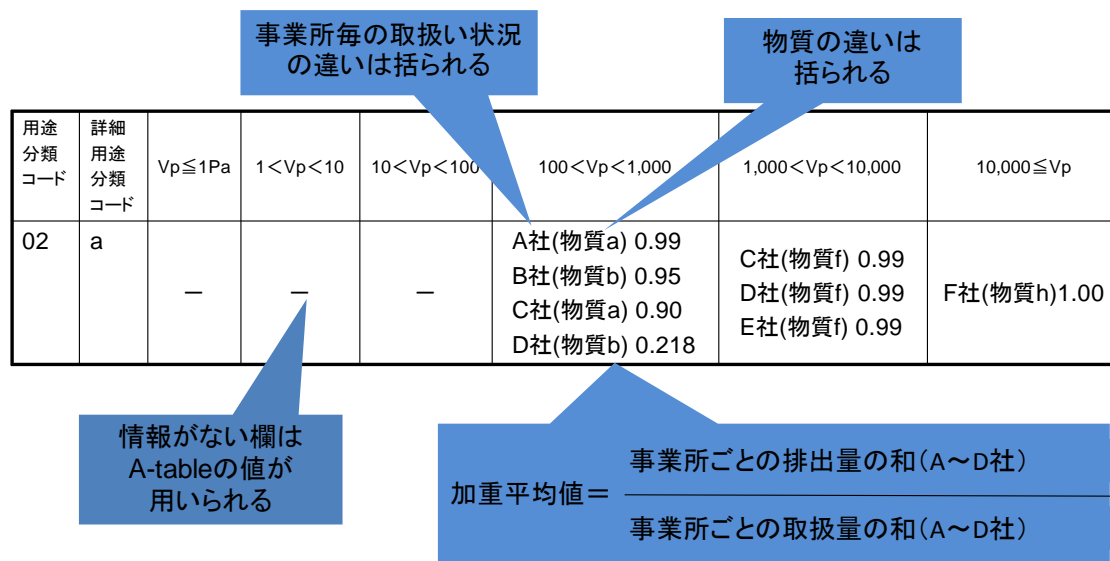
図表 IV-71 PRTR データ等の排出係数一覧表への反映方法のイメージ
