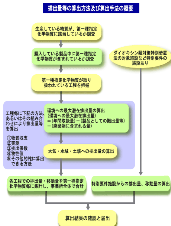
図表 IV-118 PRTR 制度における排出量の算出方法及び算出手法の概要フロー
