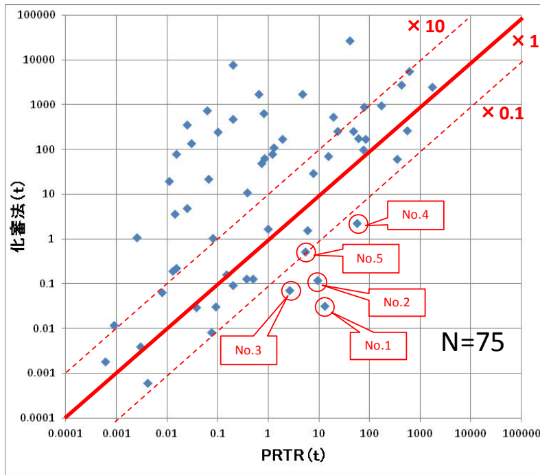
図表 IV-127 化審法推計排出量と PRTR 届出排出量最大排出源の比較検証—大気
