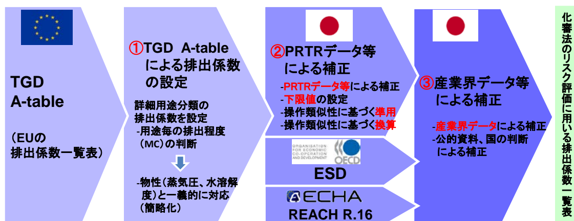
17 18 図表 IV-67 排出係数の設定方法の全体フロー
