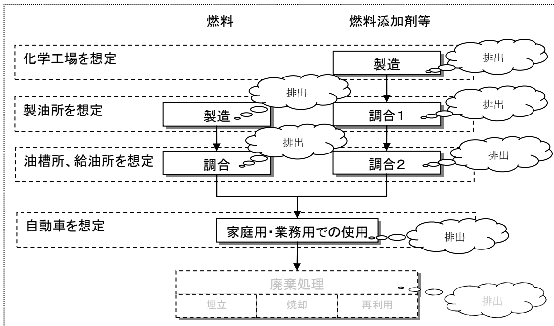
15 図表 IV-23 燃料及び燃料添加剤の優先評価化学物質のライフサイクル
