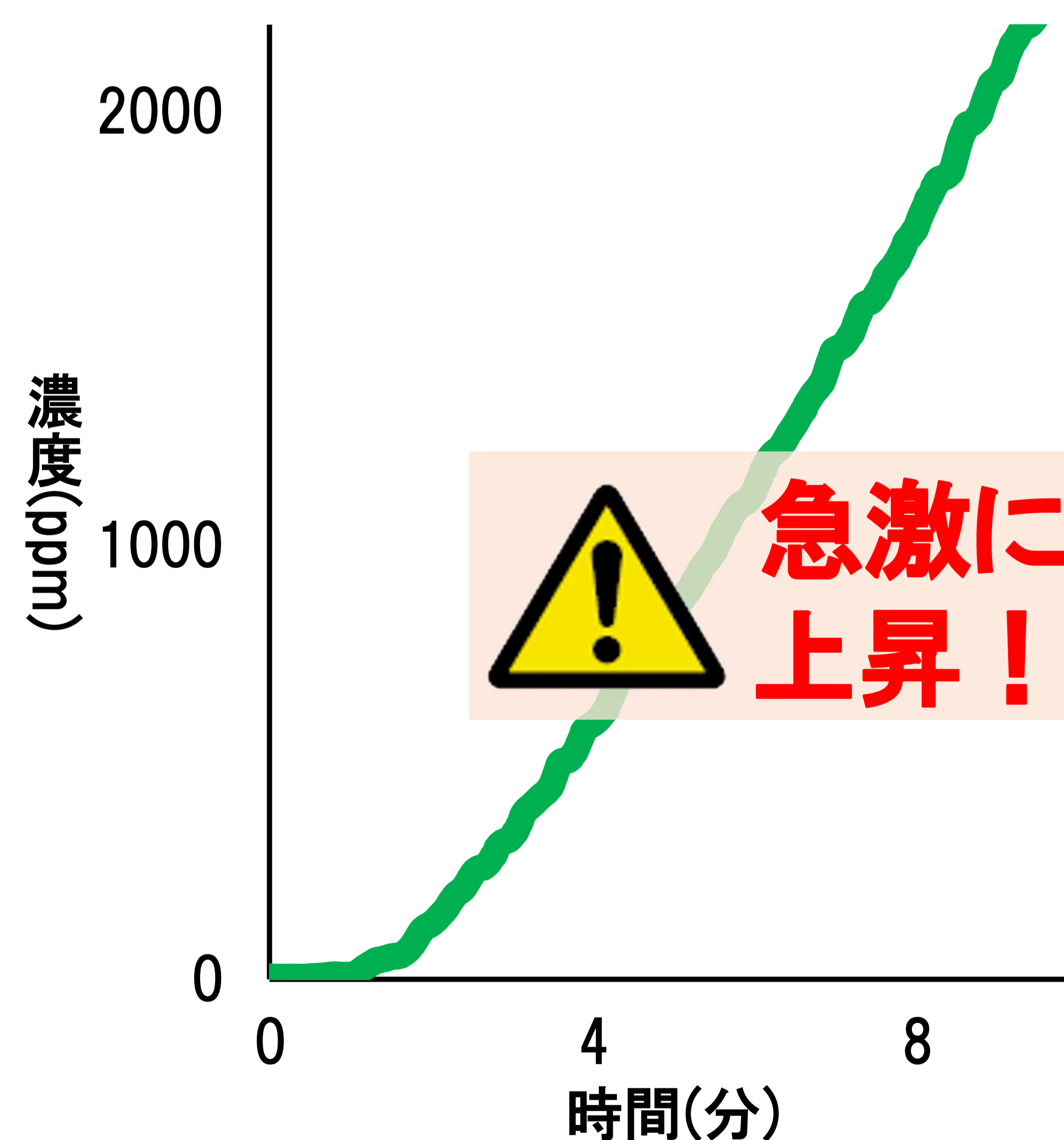
携帯発電機を屋内で使用した場合のCO濃度の変化の実験例
