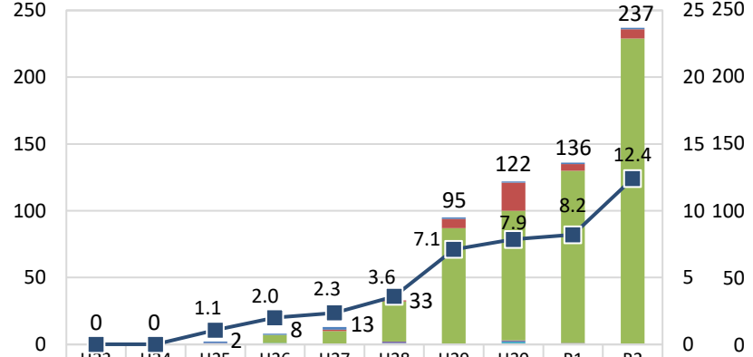
太陽電池発電所 (件) (件/100万kW)
