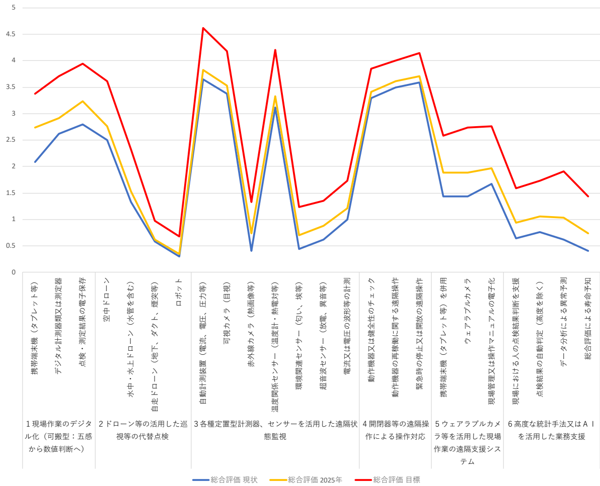
Figure 2-61 水力発電における個別技術の総合評価
