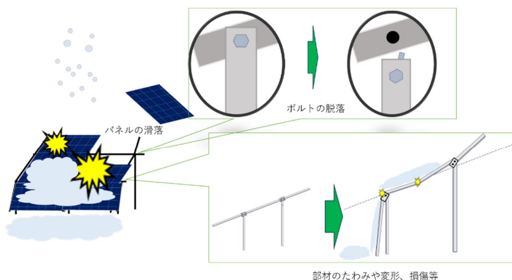
(図 5) 架台破損リスクのイメージ
