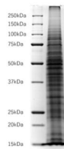
タンパク質の分離 （電気泳動）
