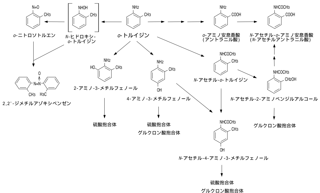
図 7-1 o -トルイジンの代謝経路 (Son et al., 1980)
